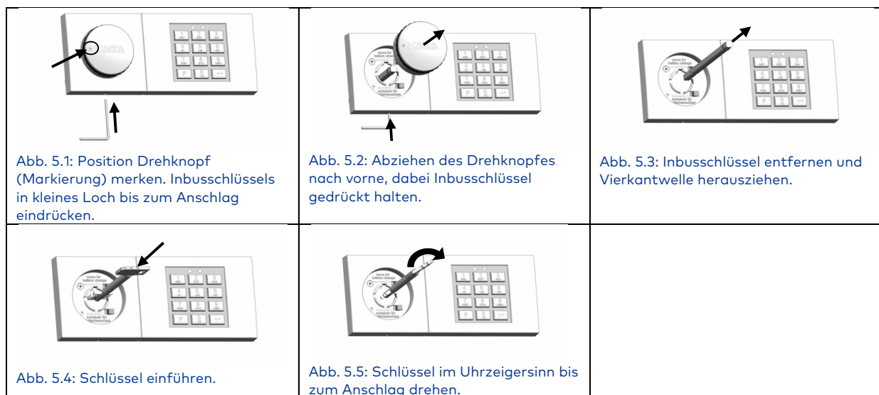
Abbildung 5: Schlüsselöffnung
